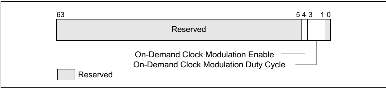
Figure 13-9. IA32_CLOCK_MODULATION MSR
