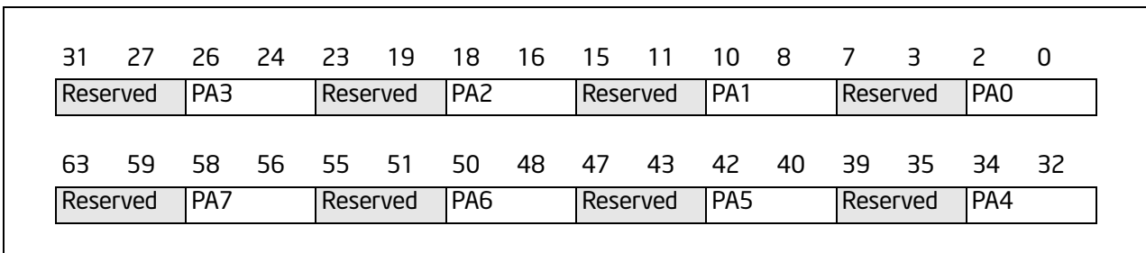
Figure 10-8. IA32_CR_PAT MSR
