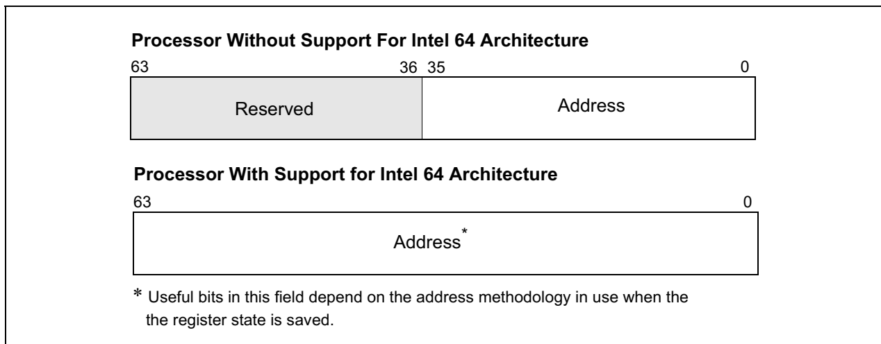
Figure 14-6. IA32_MCi_ADDR MSR
